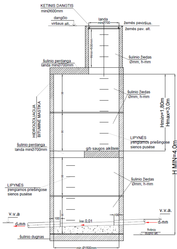
2 pav. G/B šulinio su saugos aikštele įrengimo schema
