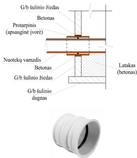
1 pav. Vamzdžio pajungimas G/B šuliniuose
