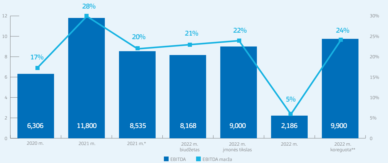
Bendrovės EBITDA (mln. Eur) rodiklio ir EBITDA maržos (proc.) kaita 2020-2022 m.
