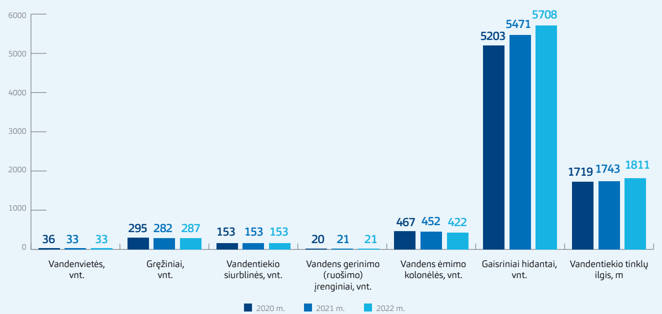
Bendrovės geriamojo vandens tiekimo procese eksploatuojama infrastruktūra 2020-2022 m.
