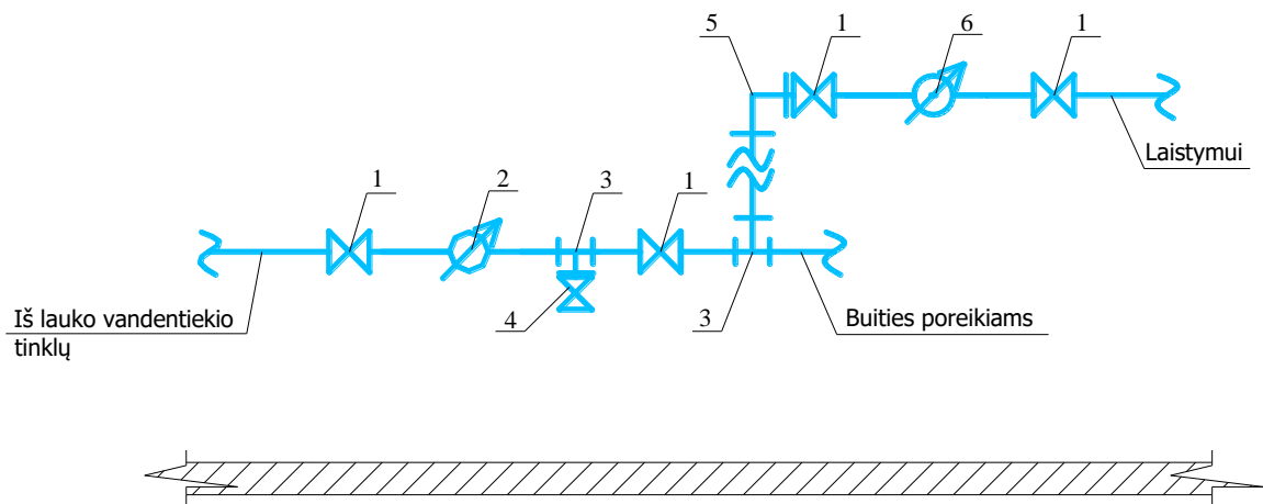
1 pav. Principinė VAM schema individualiam namui su laistymu
