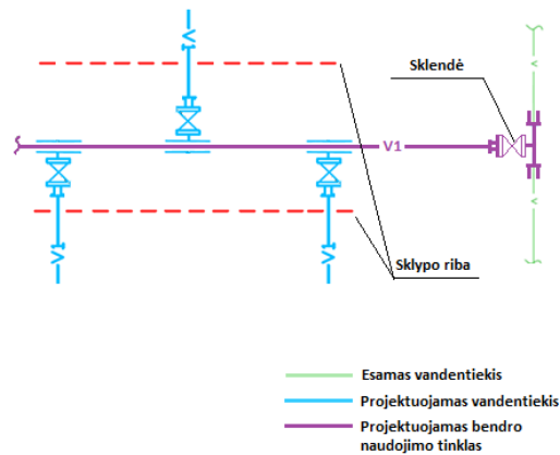
5 pav. Prisijungimo schema, kai reikalingi bendro naudojimo tinklai
