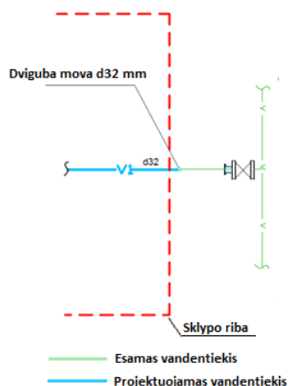
7 pav. Vienbučio individualus gyvenamojo namo prisijungimo prie vandentiekio tinklo, kai yra palikta perspektyvinė atšaka po žeme schema (standartinė prijungimo schema)
