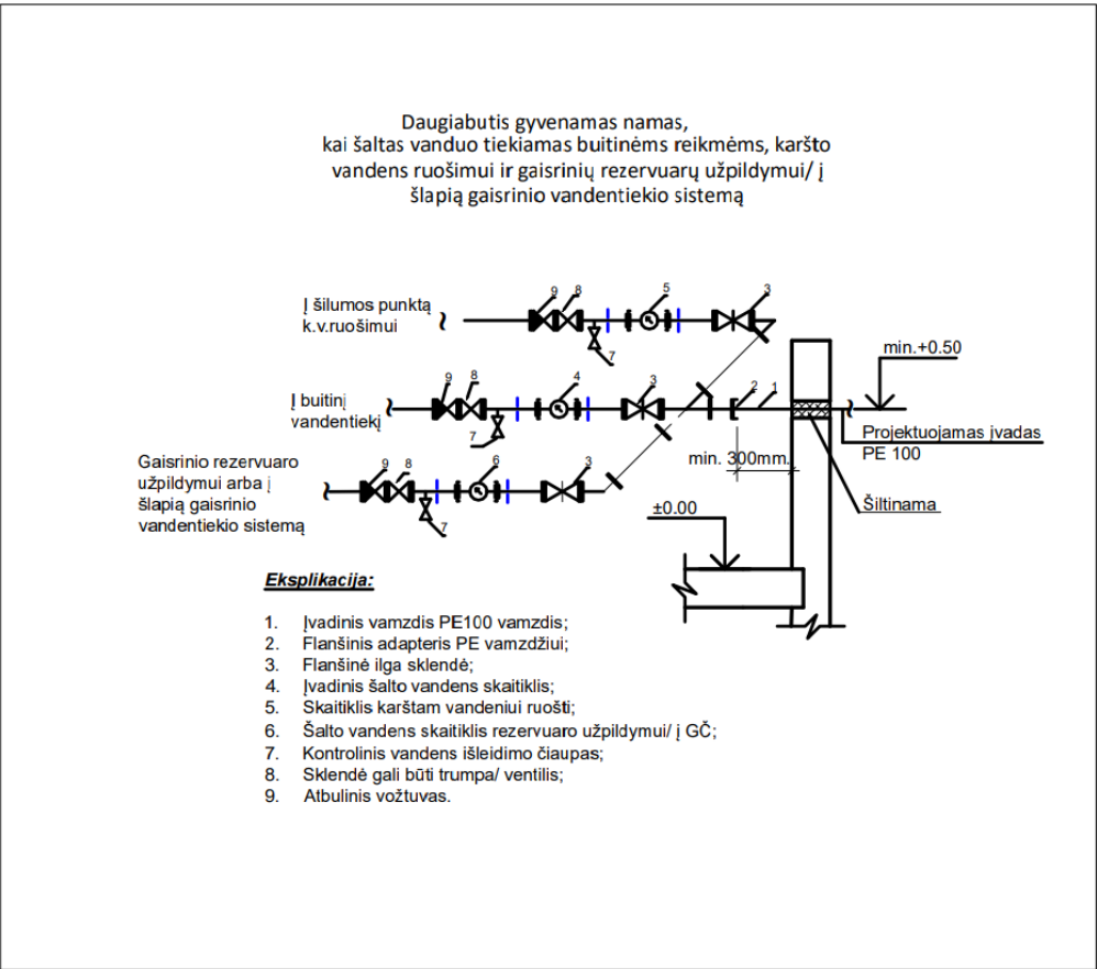
41 pav. daugiabutis gyvenamas namas, kai šaltas vanduo tiekiamas buitinėms reikmėms, karšto vandens ruošimui ir gaisrinių rezervuarų užpildymui/ į šlapią gaisrinio vandentiekio sistemą
