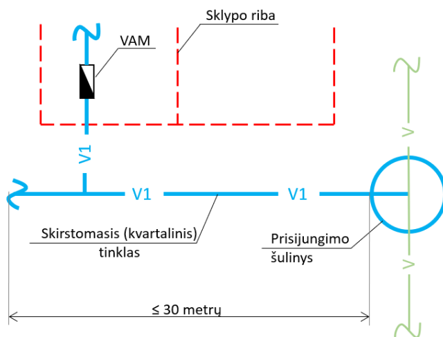
50 pav. Skirstomieji kvartaliniai tinklai, kai apskaita VAM
