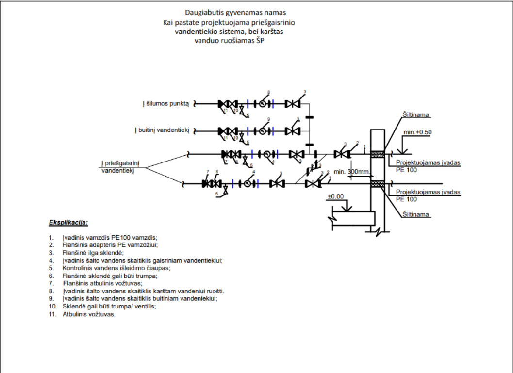
43 pav. daugiabutis gyvenamas namas, kai pastate projektuojama priešgaisrinio vandentiekio sistema, bei karštas vanduo ruošiamas ŠP
