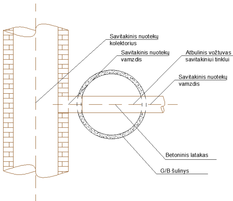
26 pav. Prisijungimo prie nuotekų kolektoriaus, montuojant šulinį prie kolektoriaus, schema
