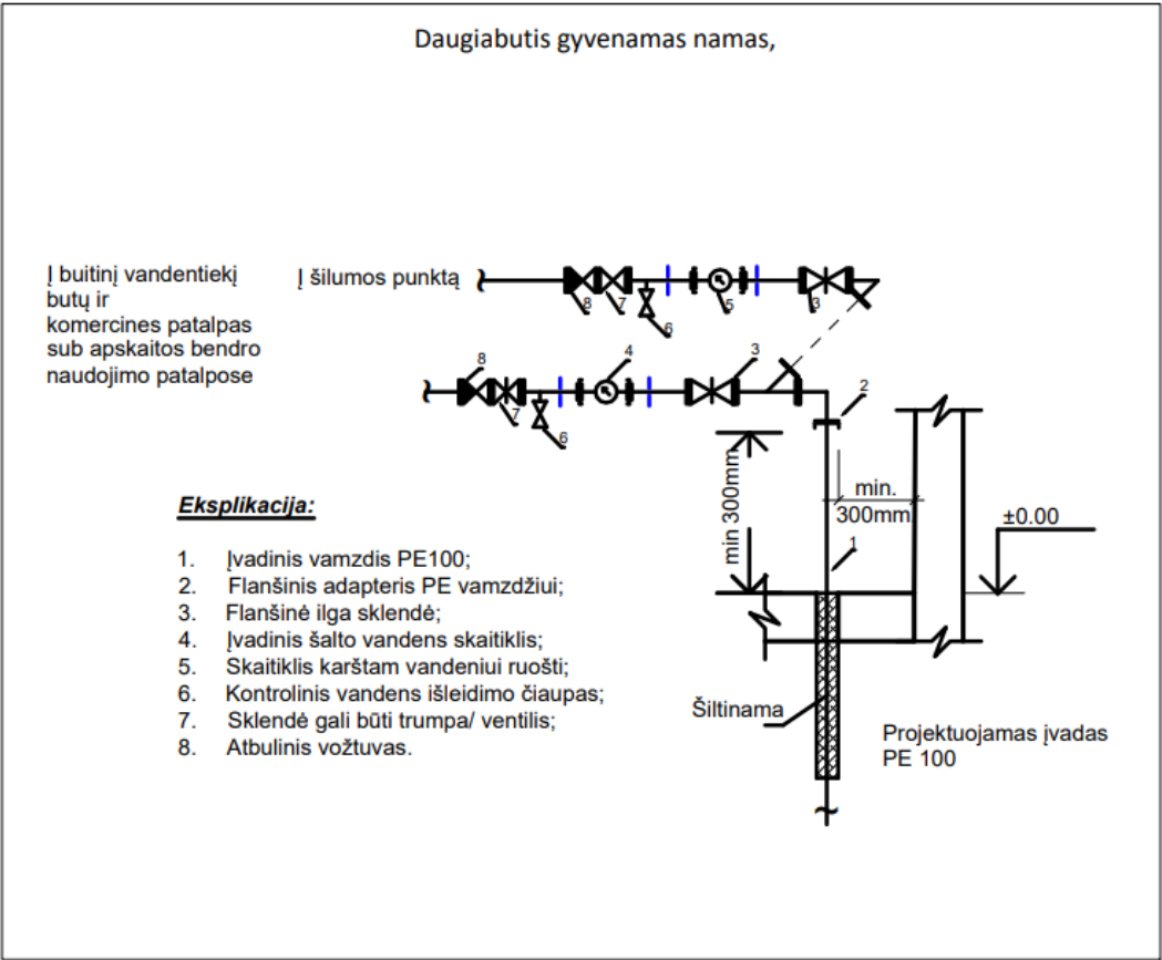
45 pav. daugiabutis gyvenamas namas
