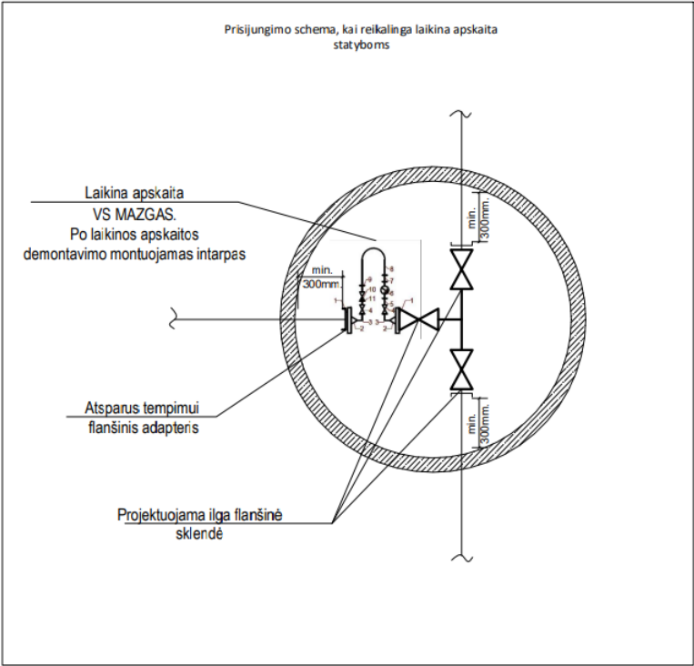
51 pav. prisijungimo schema, kai reikalinga laikina apskaita statyboms
