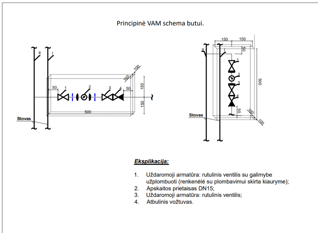
34 pav. principinė vandens apskaitos mazgo schema
