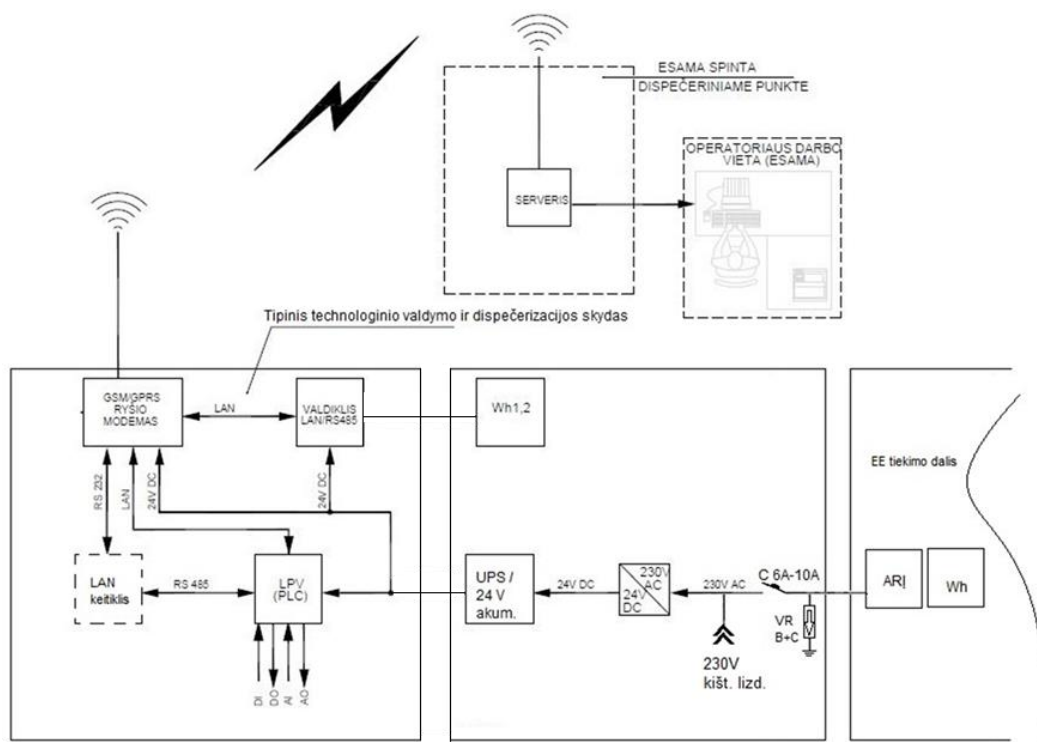
57 pav. Rekomendacinė valdymo skydo schema
