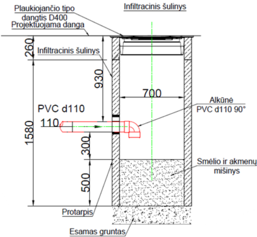
1.3 pav. infiltracinio šulinio įrengimo principinė schema
