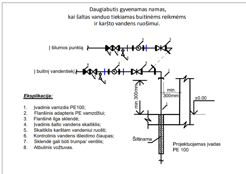
39 pav. daugiabutis gyvenamas namas, kai šaltas vanduo tiekiamas buitinėms reikmėms ir karšto vandens tiekimui
