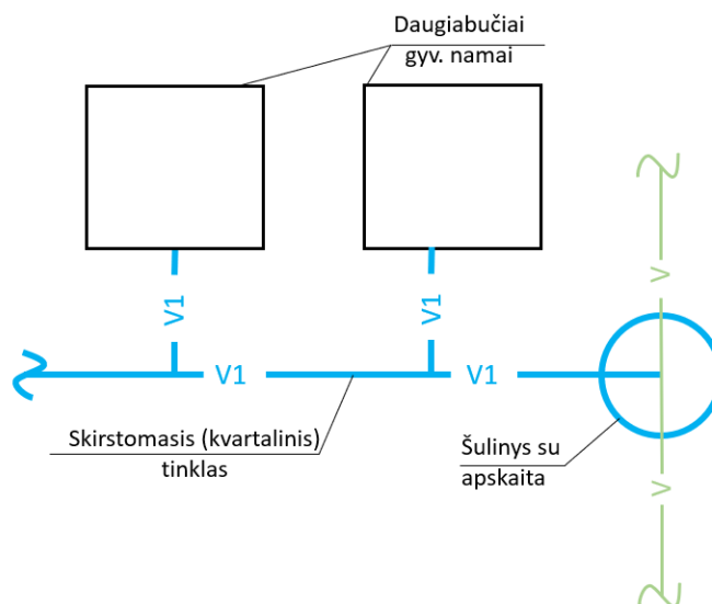
49 pav. Daugiabučių gyv. namų kvartaliniai tinklai, kai apskaita šulinyje, prisijungimo vietoje
