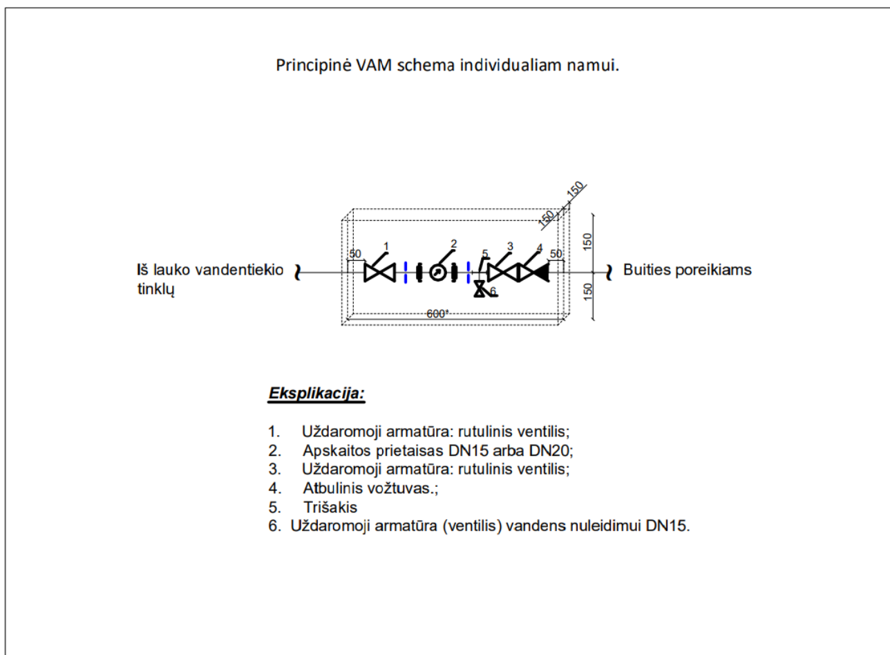
36 pav. vandens apskaitos mazgo schema individualiam namui
