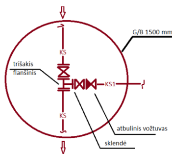
16 pav. Prisijungimo schema, kai jungiamasi prie slėginio nuotekų tinklo DN110 – 300, jungiant DN90-DN110 vamzdį
