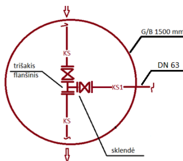
15 pav. Prisijungimo schema, kai jungiamasi prie slėginio nuotekų tinklo DN90 – 110, jungiant DN63 vamzdį
