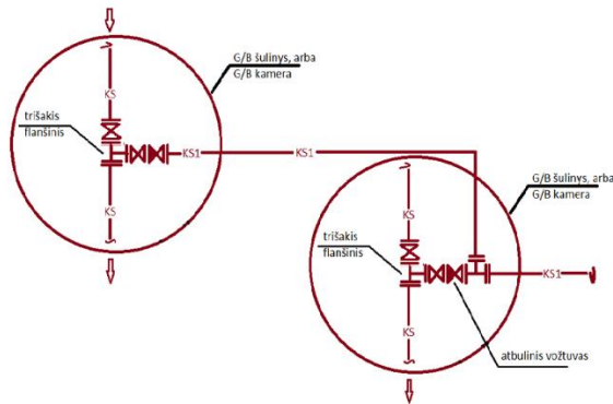
17 pav. Dviejų slėginių linijų jungimo schema
