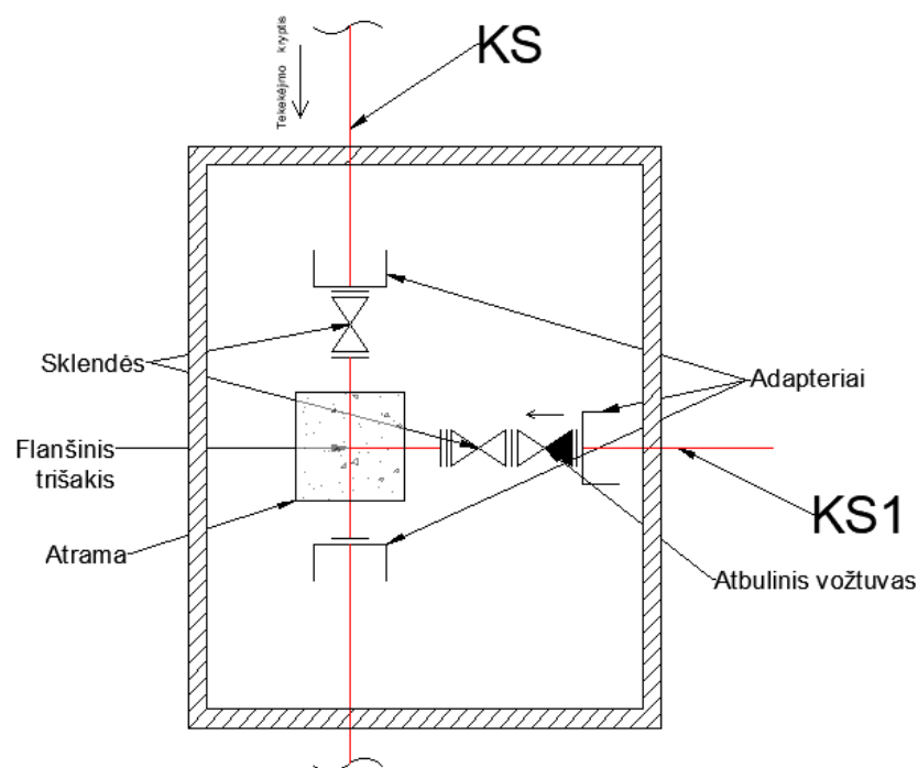
18 pav. Prisijungimo schema, kai jungiamasi prie >DN300
