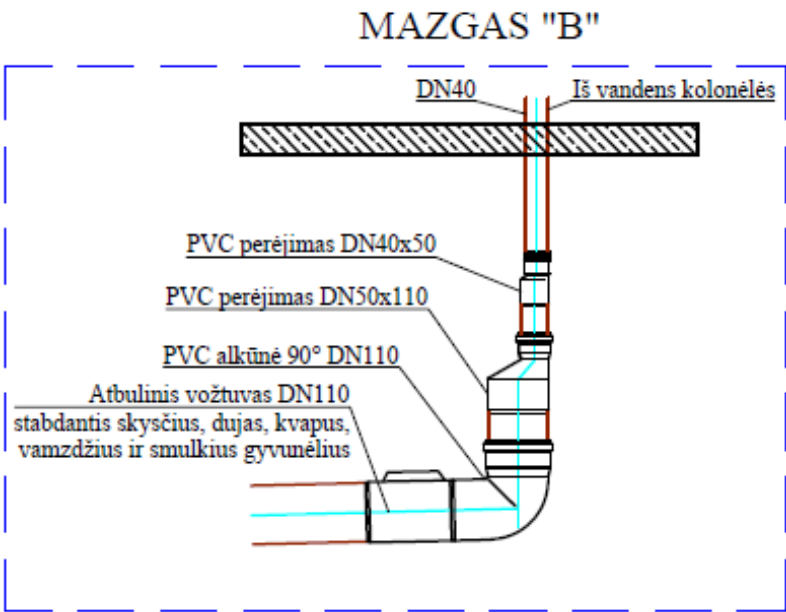
1.2 pav. perteklinio vandens nudrenavimo mazgo principinė schema
