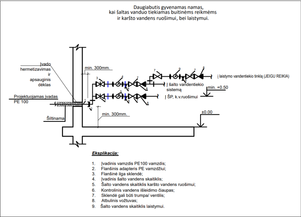
40 pav. daugiabutis gyvenamas namas, kai šaltas vanduo tiekiamas buitinėms reikmėms ir karšto vandens tiekimui, bei laistymui
