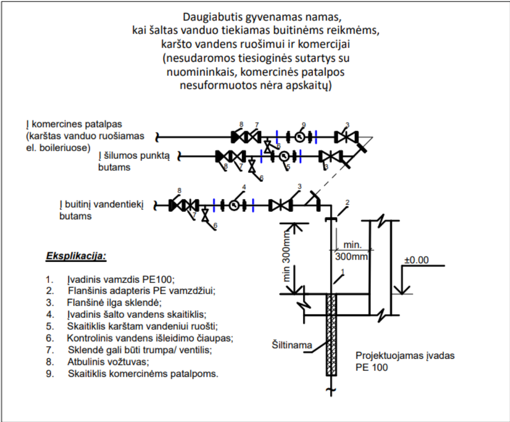
44 pav. daugiabutis gyvenamas namas, kai šaltas vanduo tiekimas buitiniams reikmėms, karšto vandens tiekimui ir komercijai
