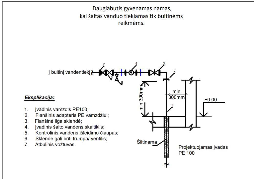
38 pav. daugiabutis gyvenamas namas, kai šaltas vanduo tiekiamas tik buitinėms reikmėms
