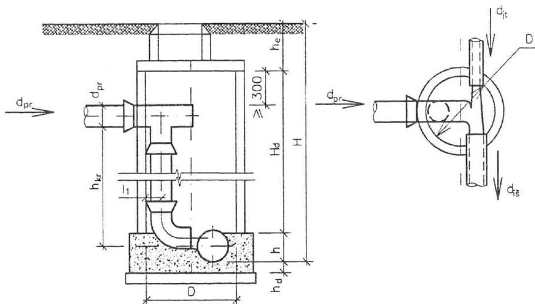
13 pav. Kritimo šulinio schema, kai reikalingas vidinis šulinys
