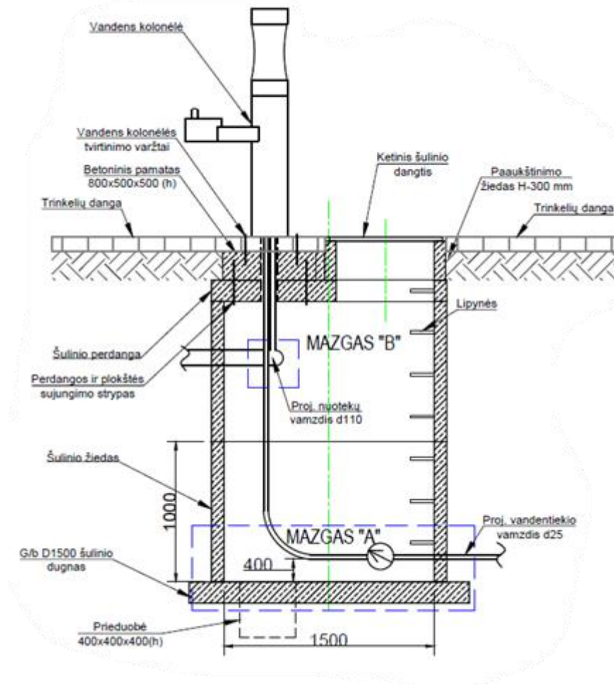
1 pav. Vandens ėmimo kolonėlės/gertuvės principinė schema
