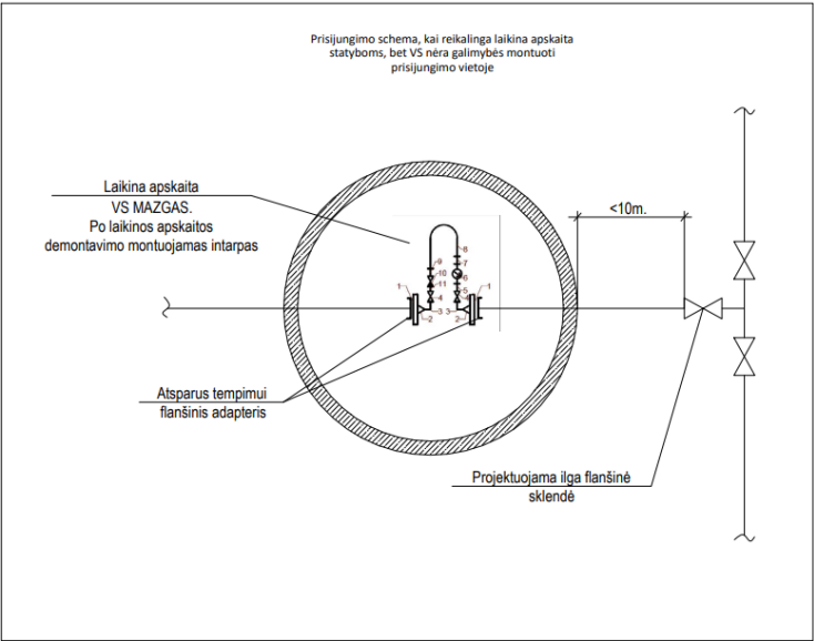
52 pav. prisijungimo schema, kai reikalinga laikina apskaita statyboms, bet VŠ nėra galimybės montuoti prijungimo vietoje
