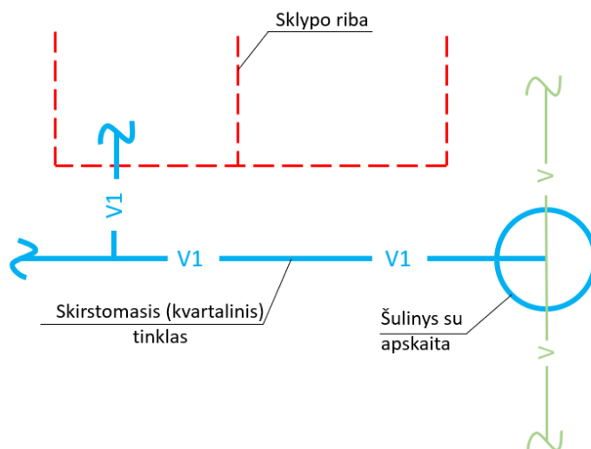
48 pav. Skirstomieji kvartaliniai tinklai, kai apskaita šulinyje, prisijungimo vietoje
