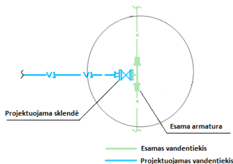
9 pav. Objekto prisijungimo prie esamo trišakio šulinyje schema (standartinė prijungimo schema)
