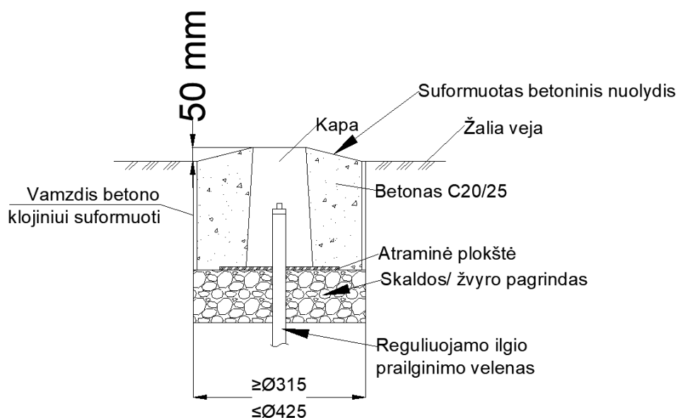
7 pav. Kapos įrengimas žalioje vejoje
