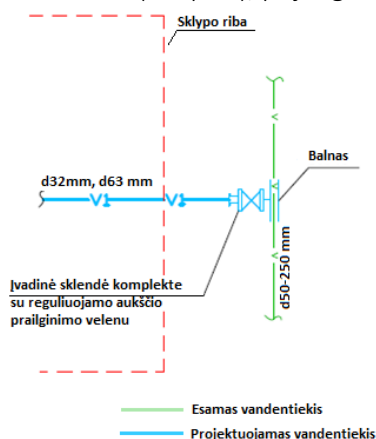
2.1 pav. Balno montavimo po žeme su uždaromąja armatūra prisijungimo schema (standartinė prijungimo schema)
