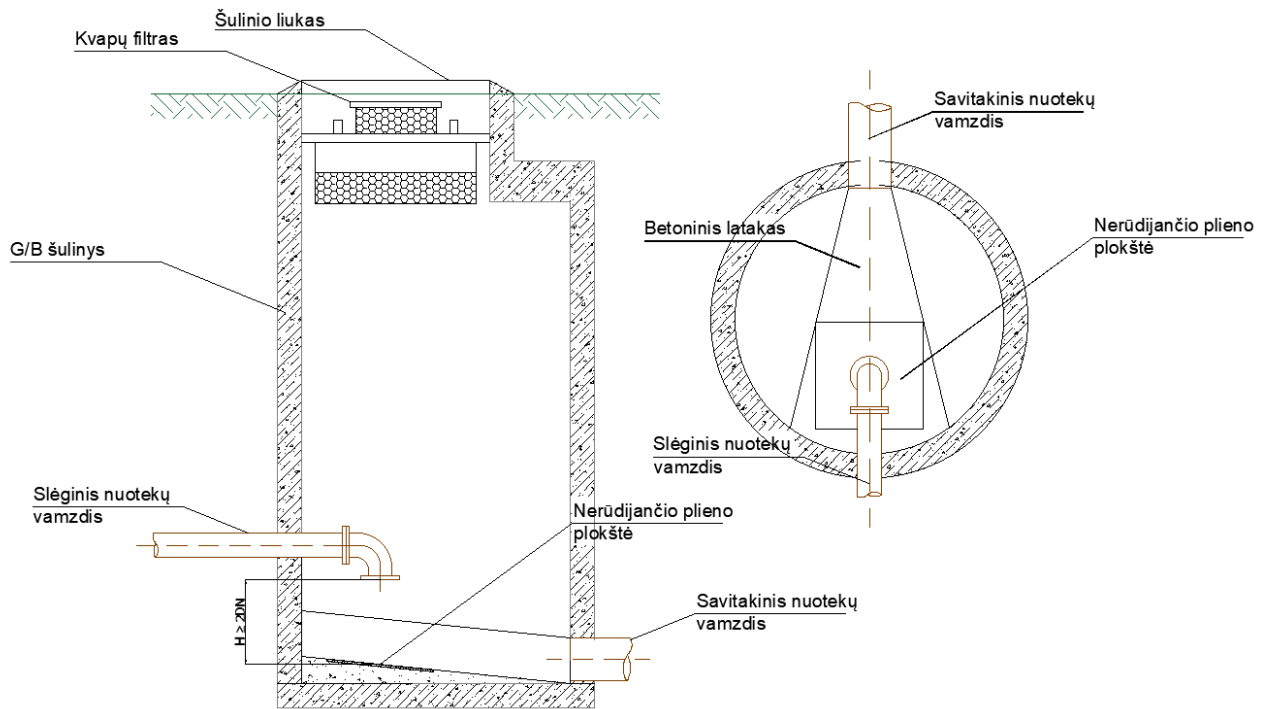
20 pav. Slėgio gesinimo šulinio principinė schema
