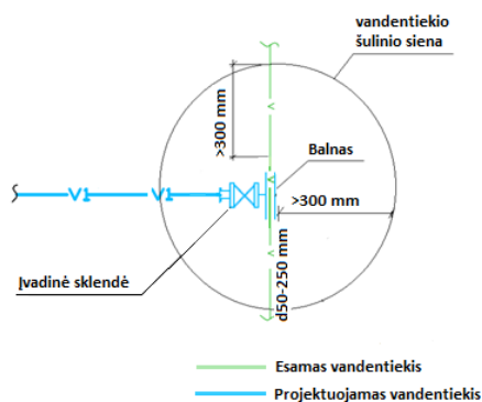
5 pav. Balno montavimo šulinyje su uždaromąja armatūra prisijungimo schema (standartinė prijungimo schema)
