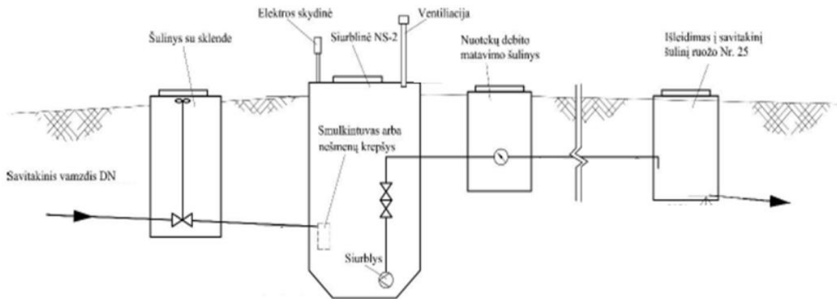
19 pav. Nuotekų siurblynės pajungimo schema
