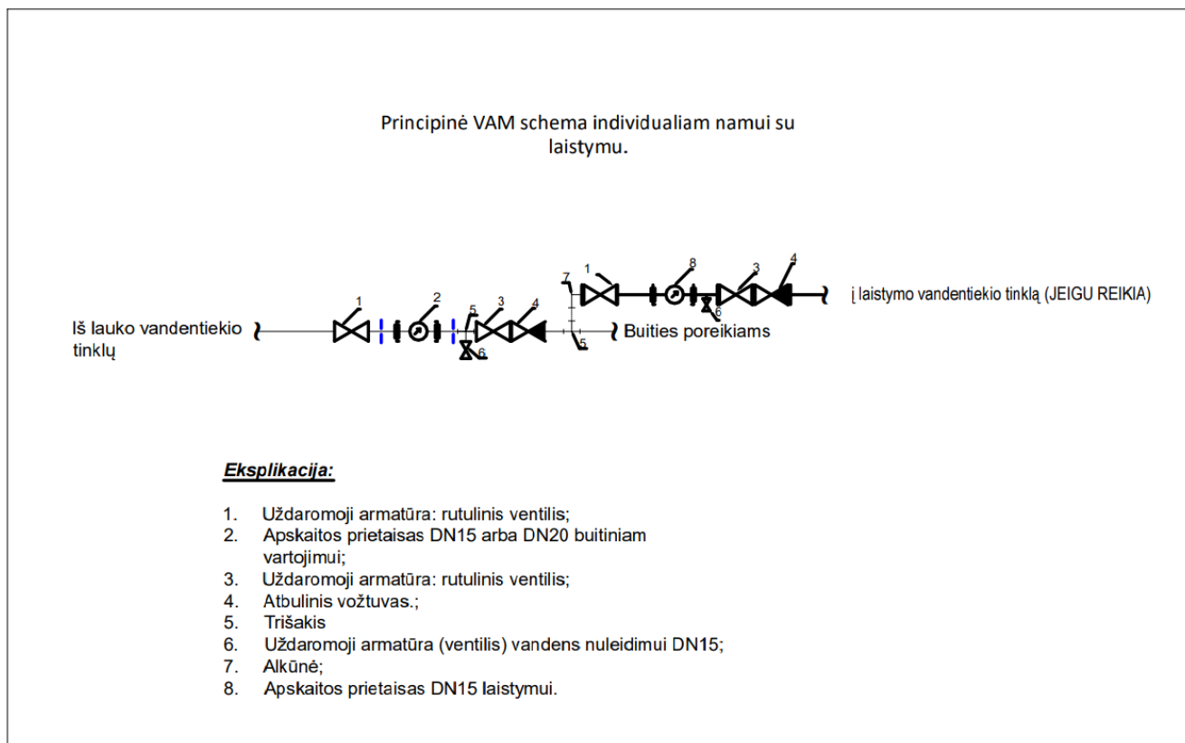
37 pav. vandens apskaitos mazgo schema individualiam namui su laistymu
