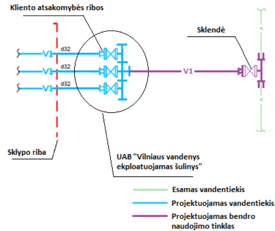
4 pav. Prisijungimo schema, kai reikalingi bendro naudojimo tinklai
