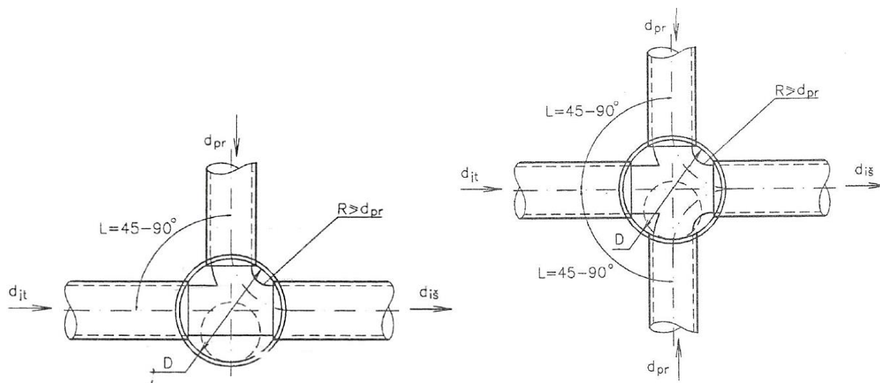
11 pav. Pasisijungimas prie savitakinio nuotekų tinklo
