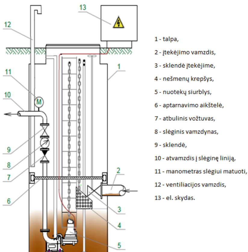
20 pav. Siurblinės schema
