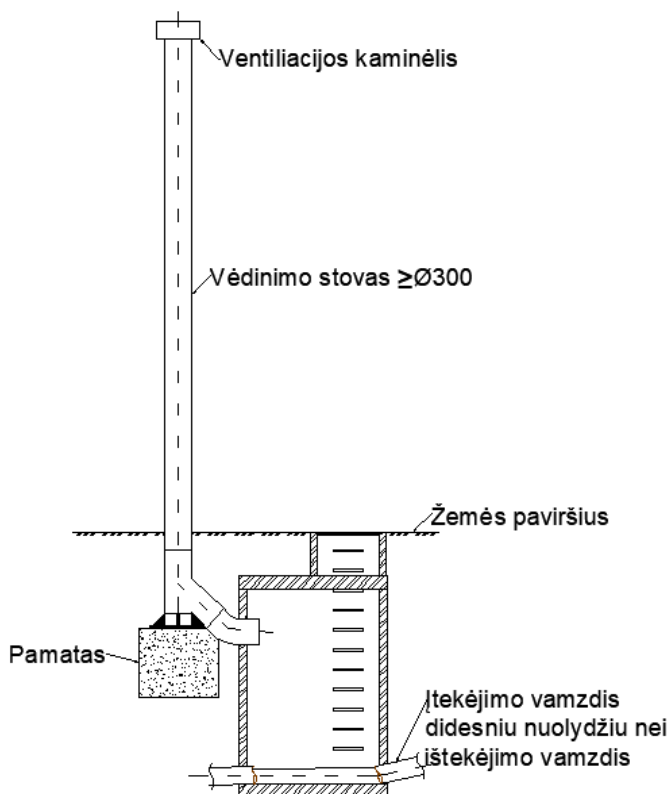
19 pav. Vėdinimo stovo šulinyje principinė schema
