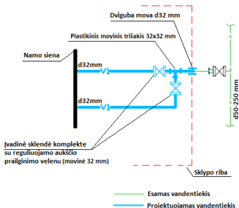
8 pav. Dvibučio gyvenamojo namo arba dvejų individualių gyvenamųjų namų prisijungimo prie vandentiekio tinklo, kai yra palikta perspektyvinė atšaka po žeme schema (standartinė prijungimo schema)
