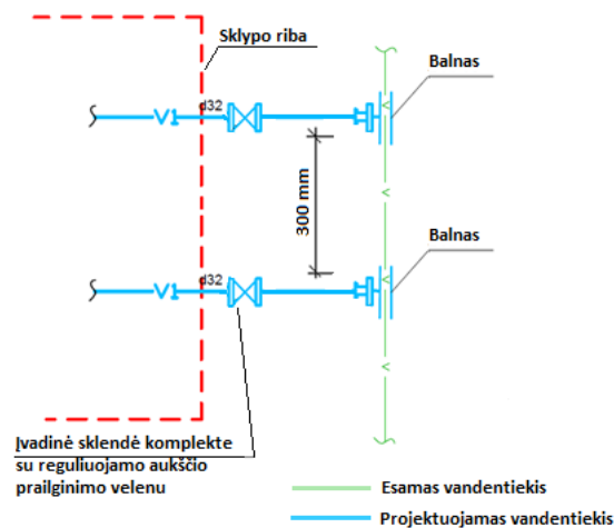
6.1 pav. Balnų montavimo po žeme be uždaroamosios armatūros, kai jungiamas dvibutis gyvenamasis namas arba du individualūs gyvenamieji namai viename sklype prisijungimo schema (standartinė prijungimo schema)
