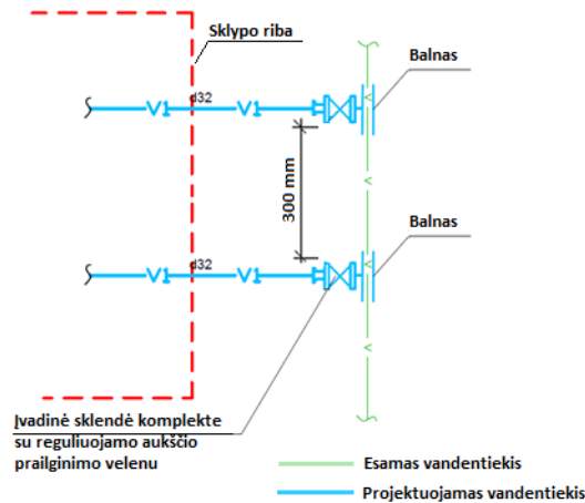
6 pav. Balno montavimo po žeme su uždarojamą armatūra, kai jungiamas dvibutis gyvenamasis namas arba du individualūs gyvenamieji namai viename sklype prisijungimo schema (standartinė prijungimo schema)
