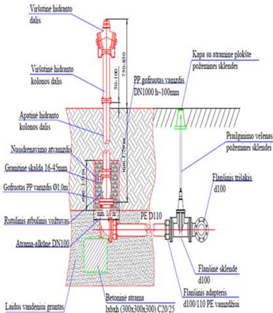
2 pav. Gaisrinio hidranto principinė schema
