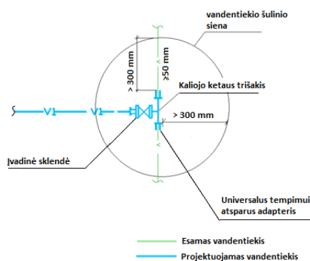
11 pav. Prisijungimo montuojant trišakį su uždaromąja armatūra šulinyje schema
