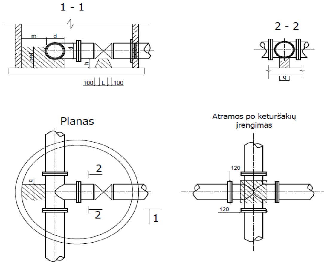
10 pav. Sklendžių atramų įrengimas
