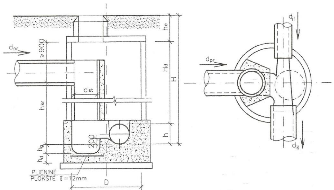
14 pav. Kritimo šulinio schema, kai reikalingas vidinis kritimo šulinys
