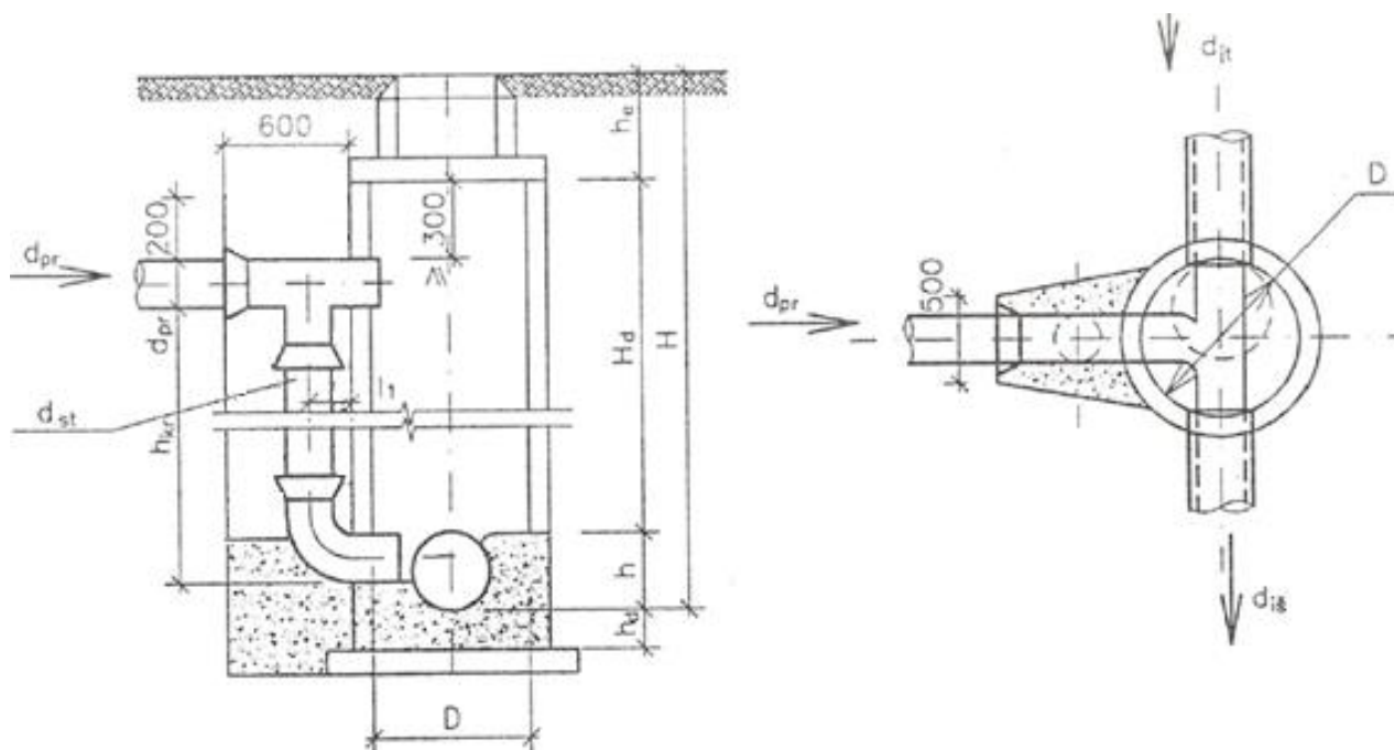
12 pav. Kritimo šulinio schema, kai reikalingas išorinis kritimo šulinys
