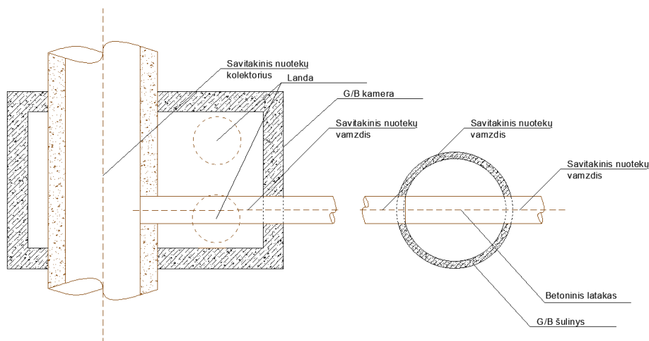
25 pav. Prisijungimo prie nuotekų kolektoriaus, montuojant šulinį ant kolektoriaus, schema
