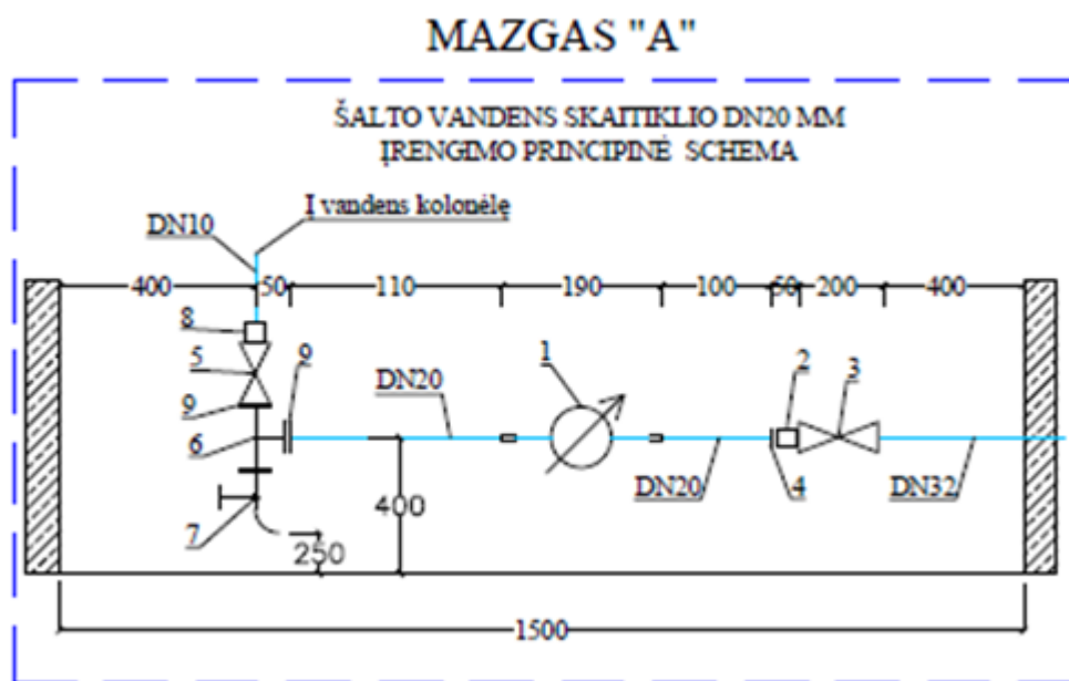
1.1 pav. vandens apskaitos mazgo šulinyje principinė schema
