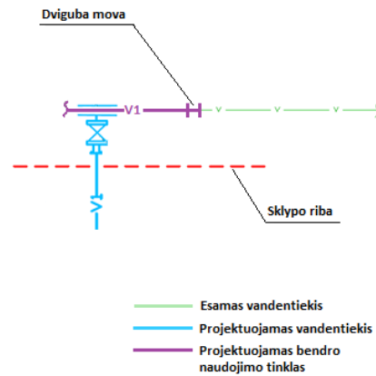
6 pav. Prisijungimo schema, kai reikalingi bendro naudojimo tinklai
