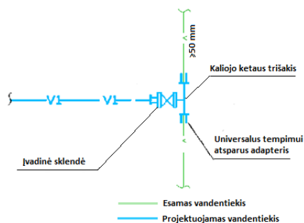
3 pav. Prisijungimo montuojant trišakį su uždaromąja armatūra po žeme schema (standartinė prijungimo schema)
