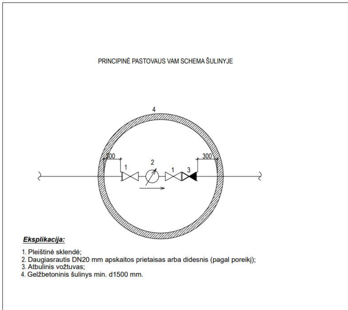
47 pav. principinė pastovaus vandens apskaitos mazgo schema šulinyje
