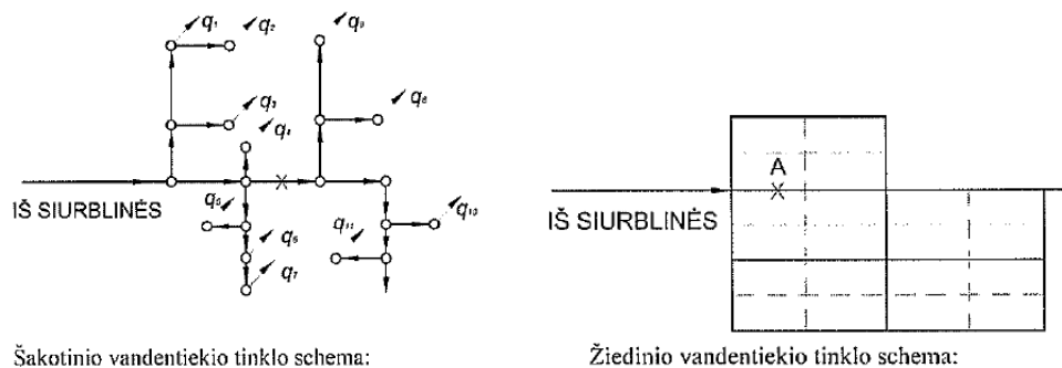
1 pav. Šakotinio ir žiedinio tinklo schemas
