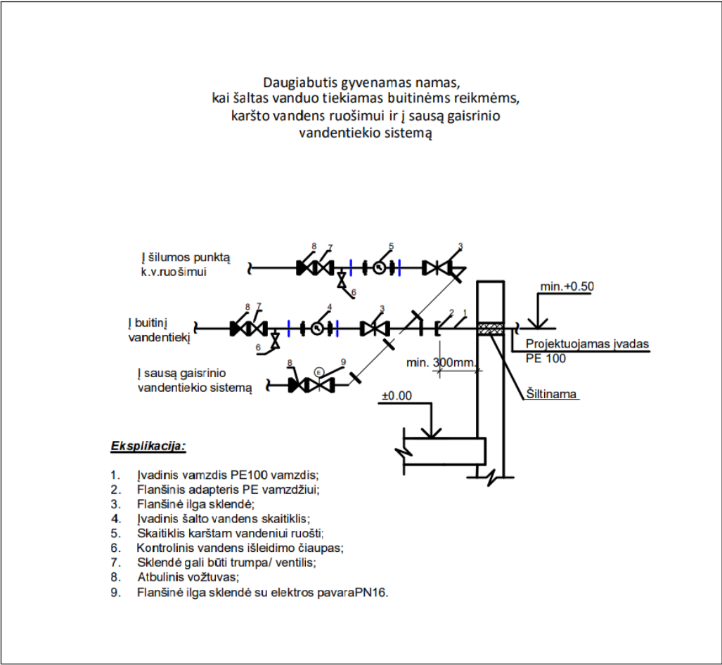
42 pav. daugiabutis gyvenamas namas, kai šaltas vanduo tiekiamas buitinėms reikmėms, karšto vandens ruošimui ir į sausą gaisrinio vandentiekio sistemą
